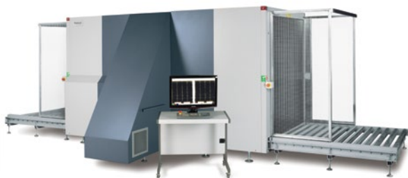
Размер досмотрового туннеля (ШИРИНА И ВЫСОТА): 1 837 x 1 800 мм
